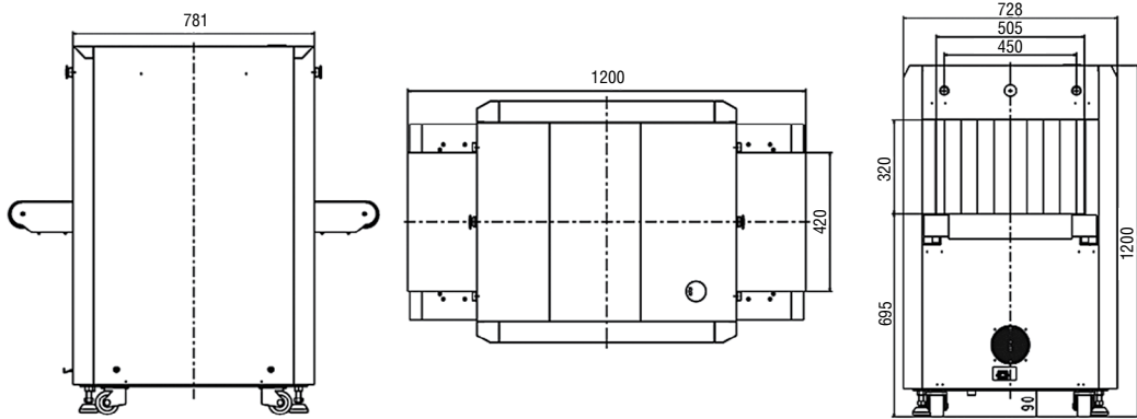
Чертеж оборудования
