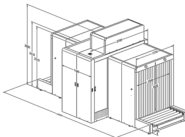
Чертеж оборудования
