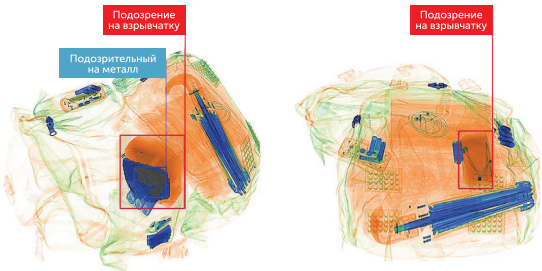
Выделение подозрительных областей изображения (автоматическая диагностика взрывчатых и наркотических веществ по Zeff)
