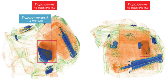
Выделение подозрительных областей изображения (автоматическая диагностика взрывчатых и наркотических веществ по Zeff)
